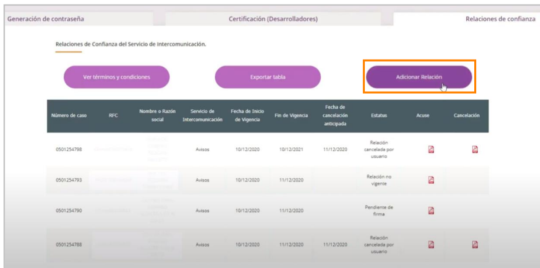
Figura 4.-Adicionar Relación.
