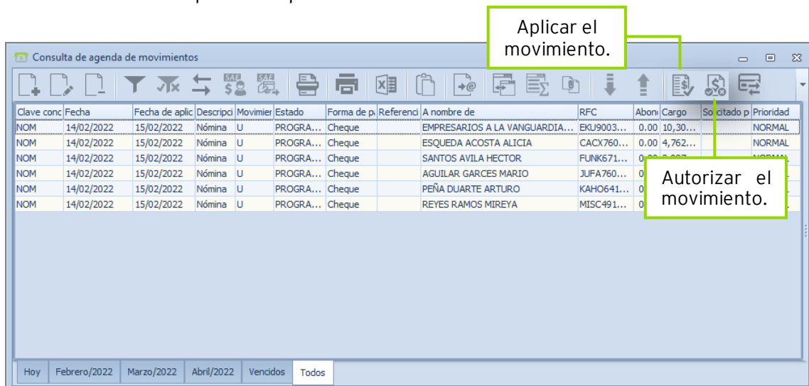
Figura 4. Agenda de movimientos bancarios en Aspel BANCO.
