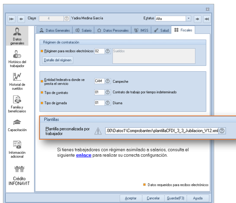
Figura 4. Configura plantilla.
