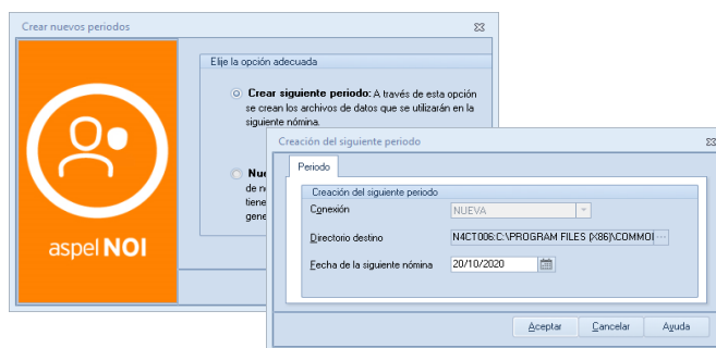
Figura 1. Crear periodo.
