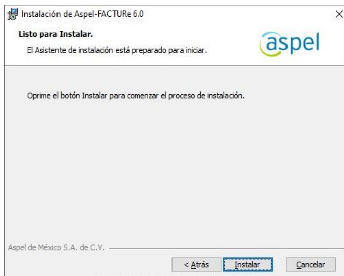
Figura 8. Instalar.
