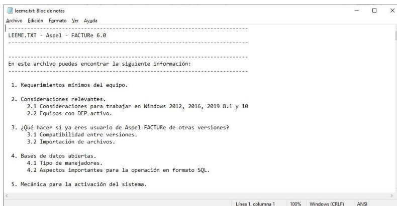
Figura 1. Archivo léeme
