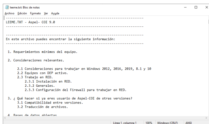
Figura 13.-Archivo léeme.
