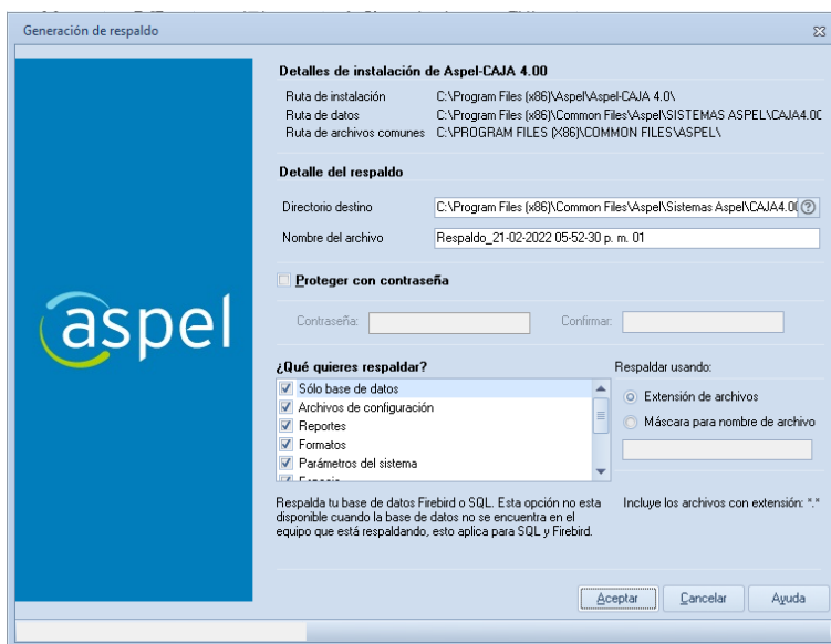
Figura 1.-Generación de respaldo de Aspel CAJA 4.0.
