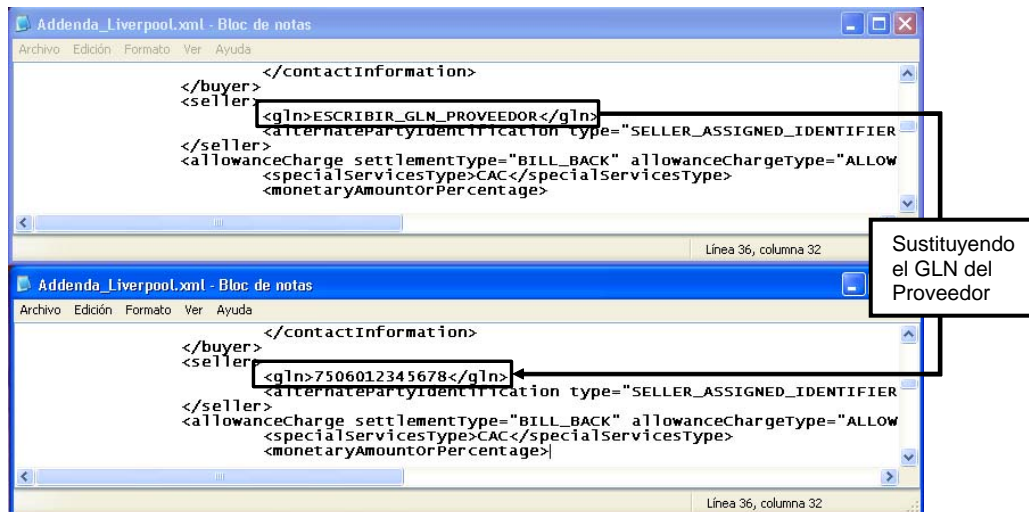
Figura 6-2. Personalizando el GLN del Proveedor.
